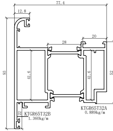
配KTGR60A10角码
