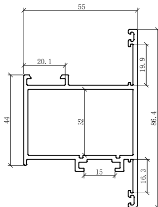
角码配KTGR1534
