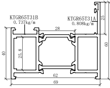
配KTGR1516角码
