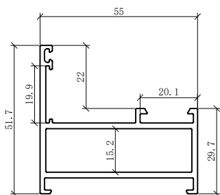
角码配KTZJ50A16
